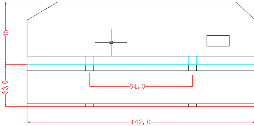
外形尺寸图
