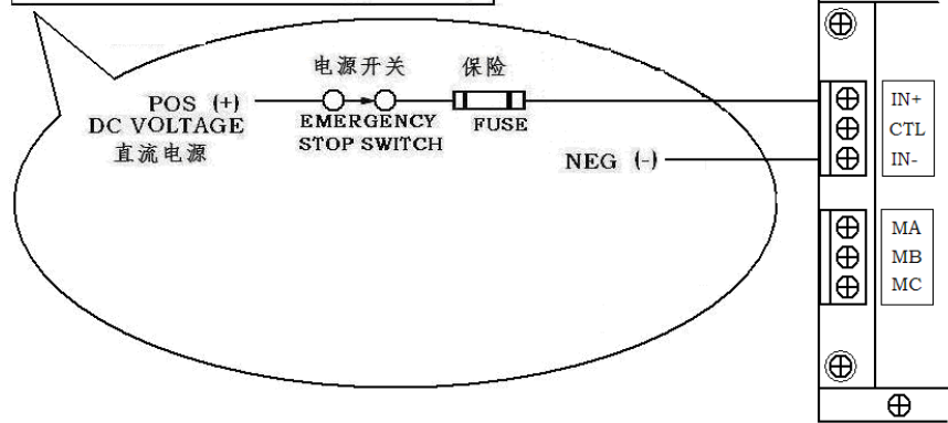
保险、电源开关的连接图
